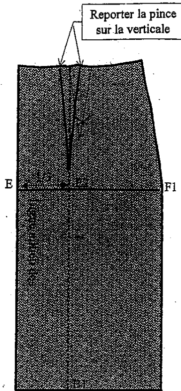
Panneau côté devant à couper 2 fois
